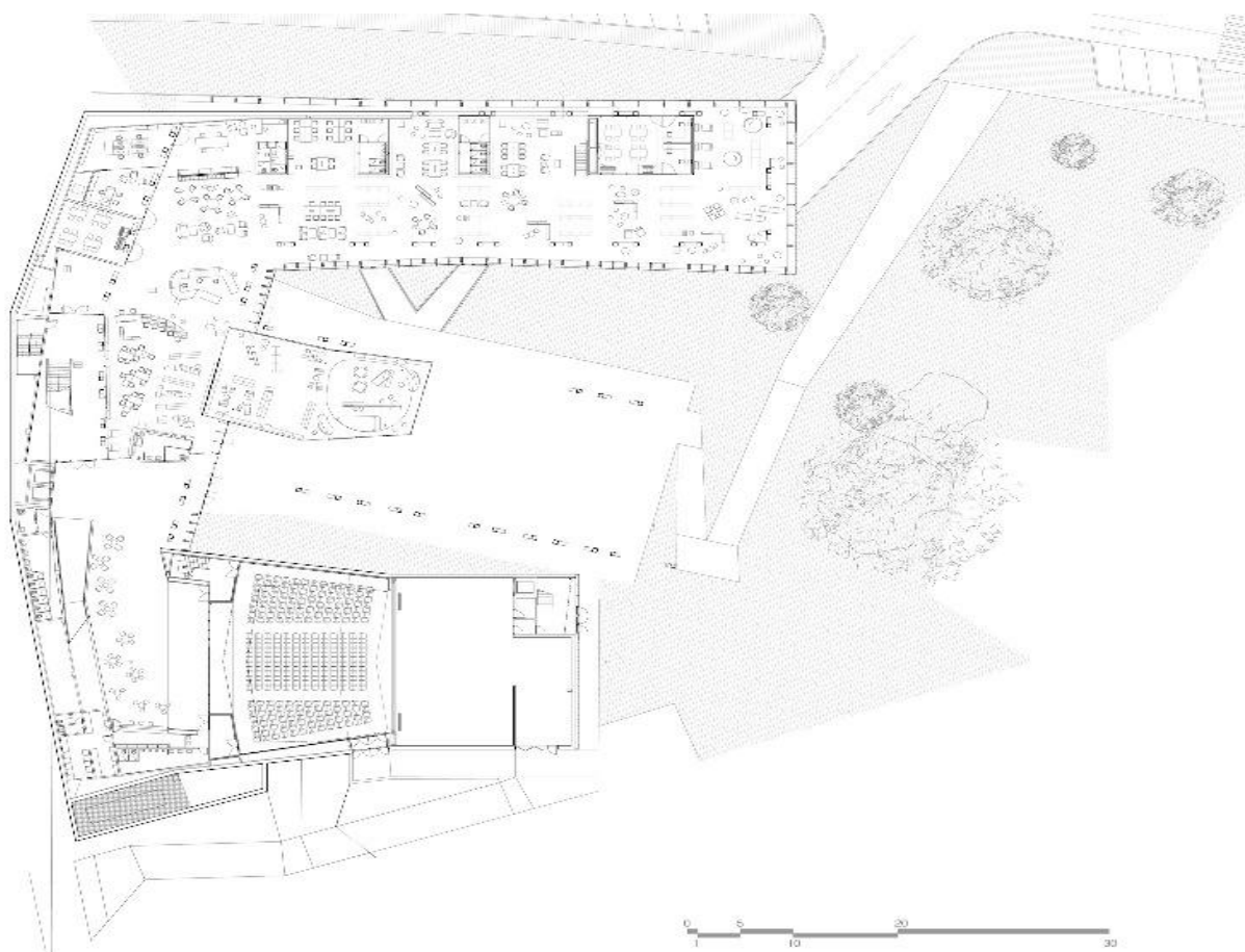
Plano del edificio Ágora
